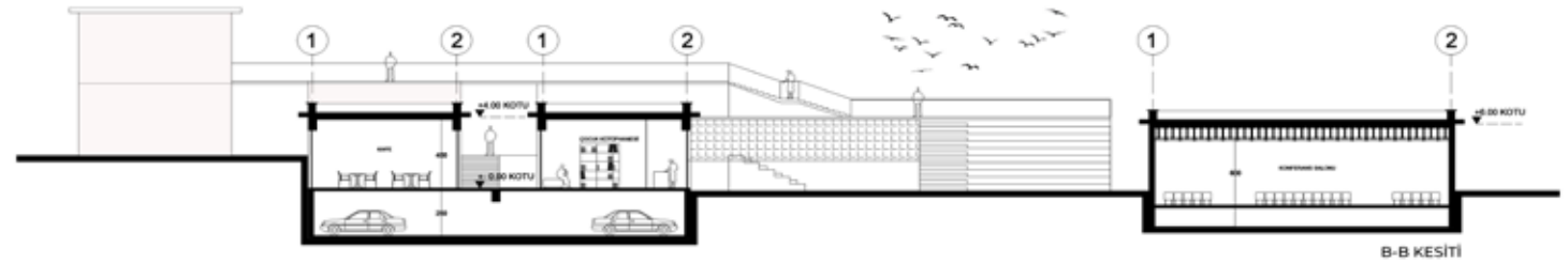
B-B KESİTİ
